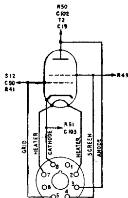
V.7. 6 V. 6 G. POWER PENTODE
